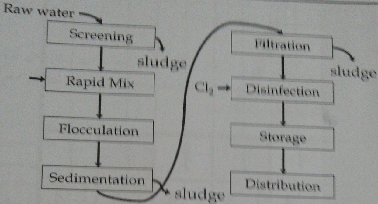
فرآیند متعارف تصفیه آب سطحی
