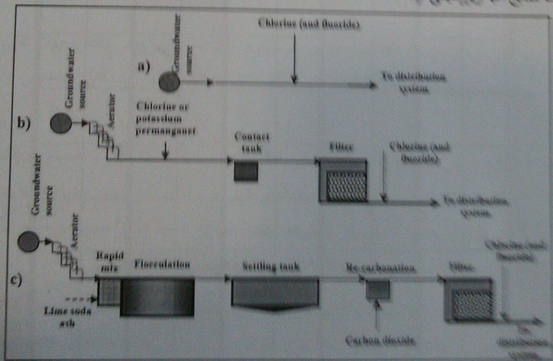
چند طرح شماتیک سیستم های متعارف تصفیه آب زیرزمینی
